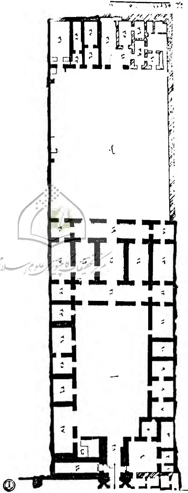
شكل رقم (٨) مخطط دار من دور الخاصة في سامراء ويلاحظ فيه الجواز الذي يفي المدخل مباشرة وعن يمينه الدملين.
